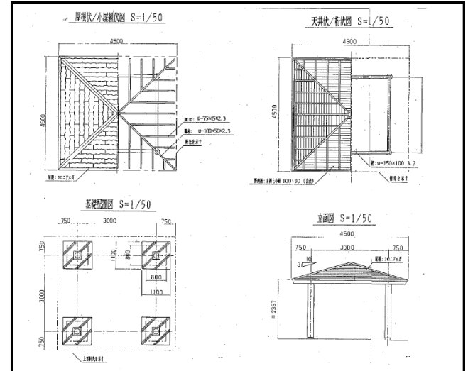
実測図面
