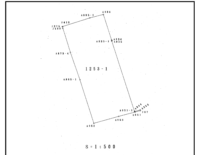
実測図面
