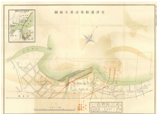
昭和八年の「宮津港修築計画平面図」
